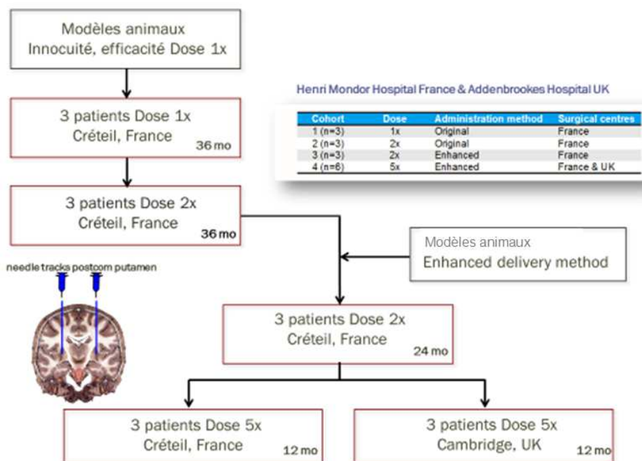
Architecture de l'essai clinique de phase I/II
